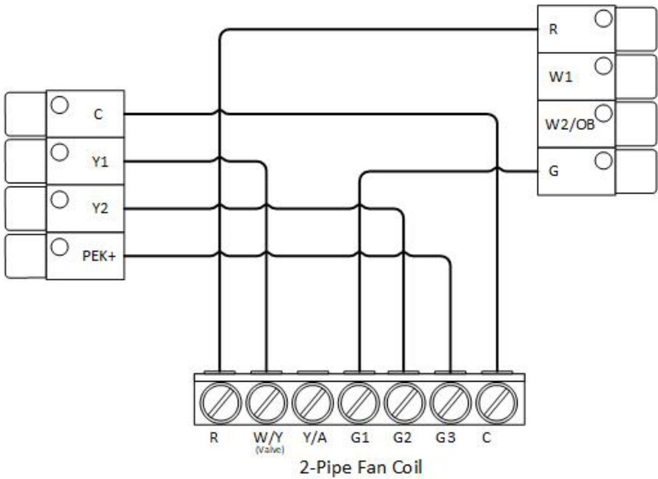
Diagram 5. Multi-speed fan 2-pipe fan coil.
