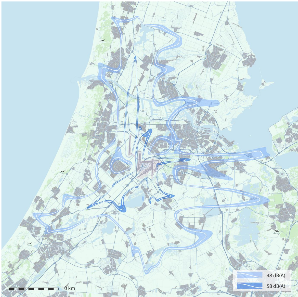
Figuur 5.1 Verwachte jaargemiddelde geluidbelasting over het etmaal Lden voor het gebruiksjaar 2017, met spreiding als gevolg van weersvariaties
