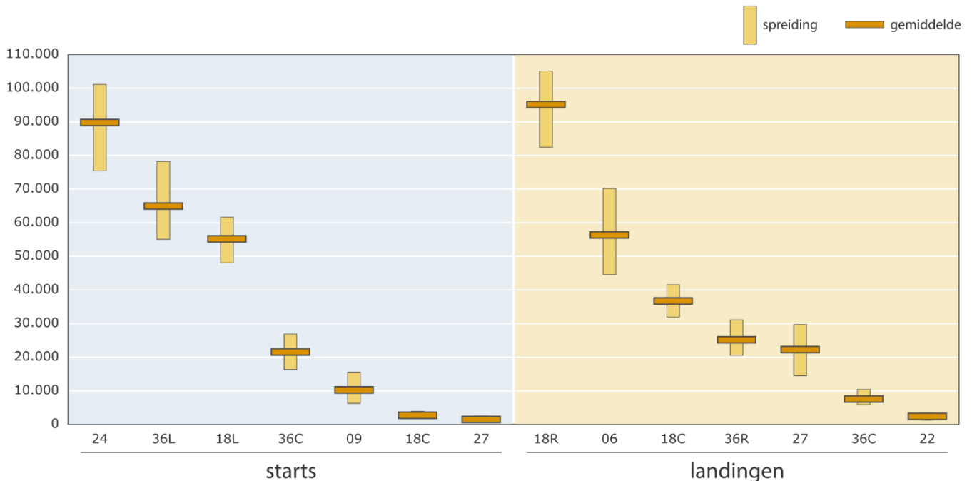
Figuur 4.3 Starts en landingen op de meest gebruikte banen Jaartotaal voor de etmaalperiode
