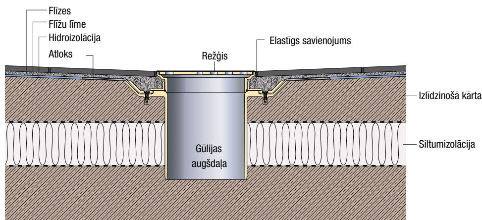
Gūlīju augšdaļa ar siltumizolāciju
