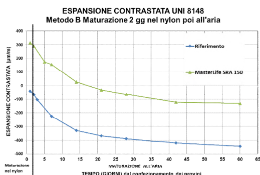
Fig. 1 Espansione contrastata UNI 8148 con MasterLife SRA 150. (Cemento CEM I 42,5 = 300 kg/m 3 , acqua = 180 l/m 3 MasterLife SRA 150 = 20 kg/m 3 ; inerti = 1975 kg/m 3 ).
