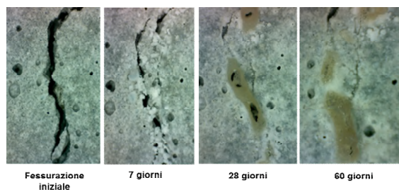
Trattamento in acqua
