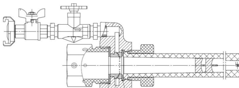
Schéma 14 : Buse de projection avec mélangeur statique, et vanne pointeau afin de réguler l'apport d'eau
