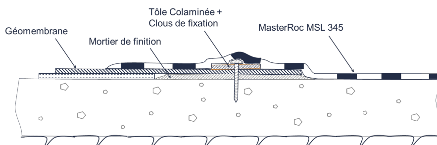
Schéma 22 : Section illustrant la disposition de l'interface entre la géomembrane PVC et le MasterRoc MSL 345 projetée.
