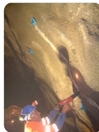
Photo 6 : Installation des tuyaux et demi coques
