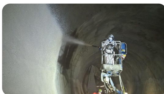
Photo 16 : Plateforme de projection appropriée
