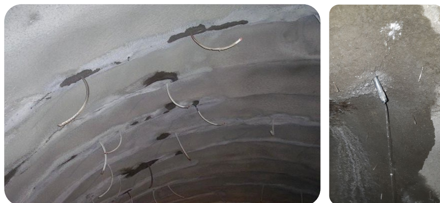
Photos 11 : Système de drainage - trous de 10 mm de diamètre contenant des injecteurs avec tuyaux en PVC, avant application du MasterRoc MSL 345 & Photos d'un injecteur utilisé comme un drain.
