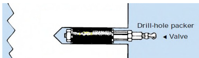
Schéma 9 : Injecteur mis en place
