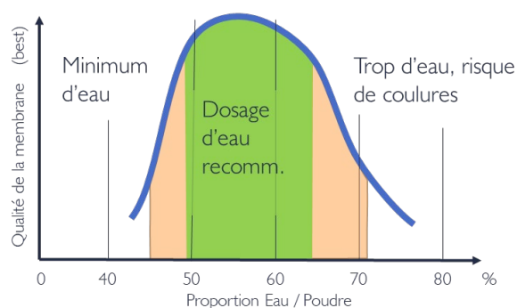
Schéma 19 : Addition d'eau recommandée
