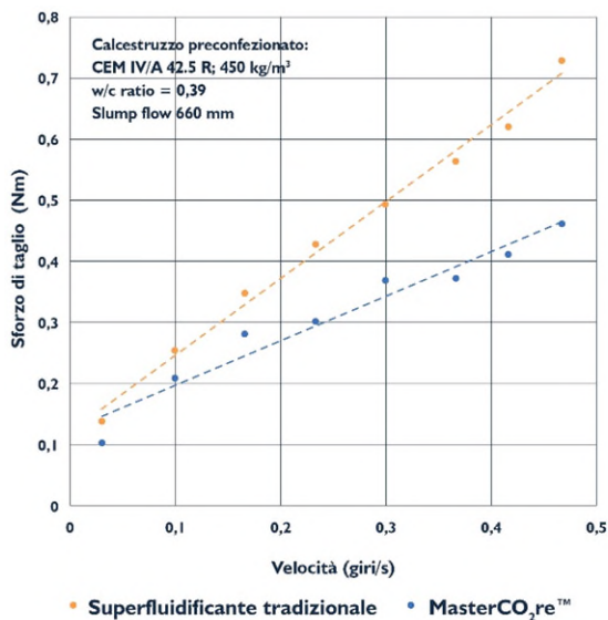
Fig. 1: Prestazioni reologiche del calcestruzzo con MasterCO 2 re 3400 (Bingham ottenuto con reometro Reiner – Rivlin)
