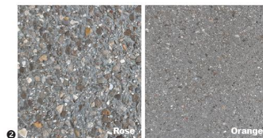
2 Aspect après lavage d'un béton en ciment gris ( D_{max} = 14 \text{ mm} ) avec MasterFinish SRT 500 Rose et Orange
