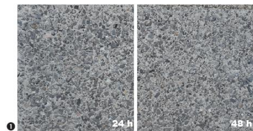
1 Aspect après lavage d'un béton en ciment blanc ( D_{max} = 14 \text{ mm} ) avec MasterFinish SRT 500 Rose à + 35°C et différentes échéances
