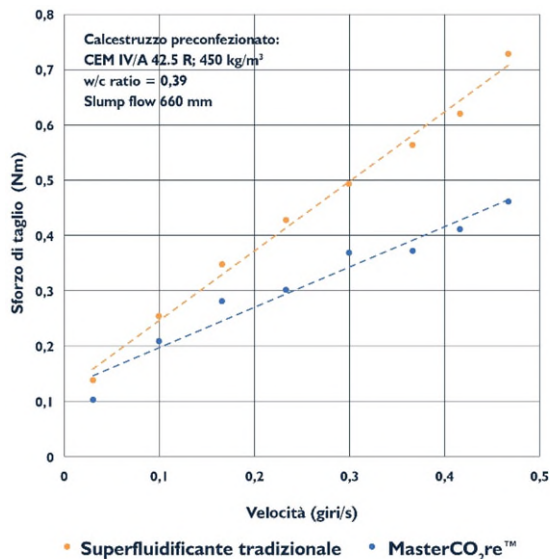
Fig. 1: Prestazioni reologiche del calcestruzzo con MasterCO 2 re 3402 (Bingham ottenuto con reometro Reiner – Rivlin)
