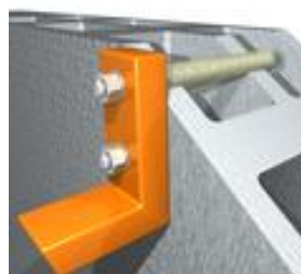
Fijación en bloques huecos
