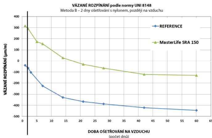
Obr. č. 1: Vázané rozpínání podle normy UNI 8148 s výrobkem MasterLife SRA 150.
