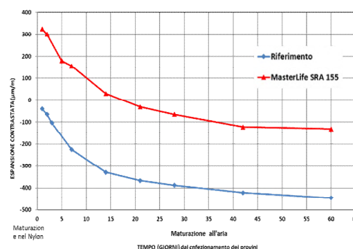
Fig. 1 Espansione contrastata UNI 8148 con MasterLife SRA I55. (Cemento CEM I 42,5 = 300 kg/m 3 , acqua = 180 l/m 3 MasterLife SRA I55 = 20 kg/m 3 ; inerti = 1975 kg/m 3 ).
