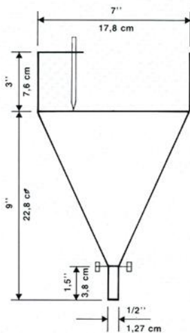
Fig. 3 – Medidas de Flow-Cone
