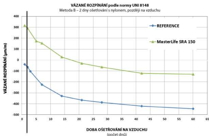
Obr. č. 1: Vázané rozpinání podle normy UNI 8148 s výrobkem MasterLife SRA 150.
