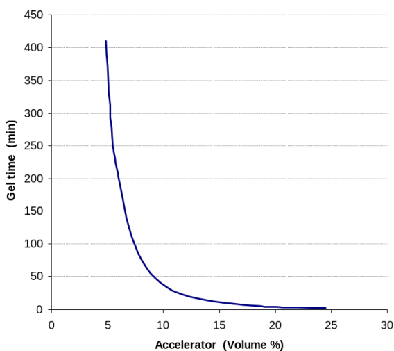
Figura 1: Gel Time con varias dosificaciones de acelerador. Valores a 20° C
