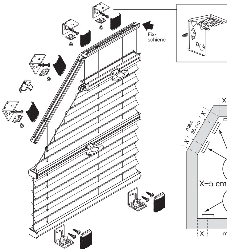
Trägermontage für schmale Fixschiene
