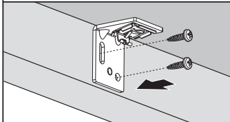
Trägermontage Schiene unten
