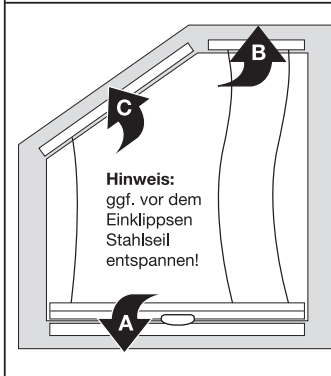
Stahlseilspannung
