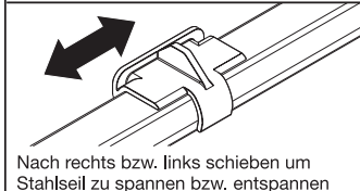
Stahlseilspannung
