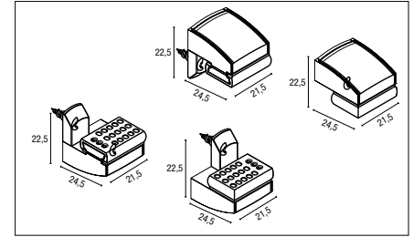
Kunststoffträger - Paar Art. Nr. 15.7999
