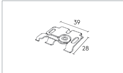
Deckenträger (oben) Art. Nr. 15.5373
