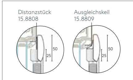
Bei runden Glasleisten: mitgelieferten Ausgleichskeil verwenden!
