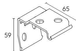
Universalträger Art. Nr. 16.6813
