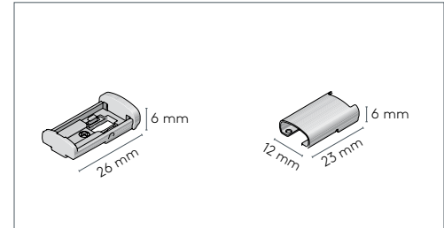
Anschraubteil: Art. Nr. 15.6456
