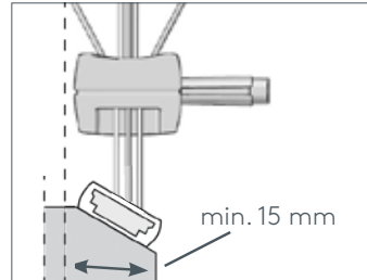
Schnitt Glasleiste mit Spannschuh und Unterschiene min. 15 mm
