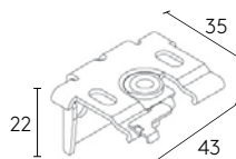
Wandträger Art. Nr. 15.5372
