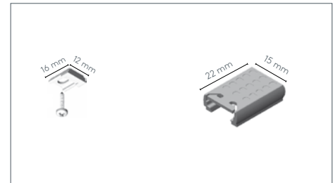
Anschraubteil: Art. Nr. 15.7828
