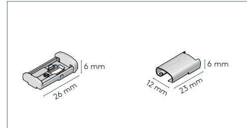
Anschraubteil: Art. Nr. 15.6456 Schnurspannerabdeckung: Art. Nr. 15.6457 mit Magnetfunktion
