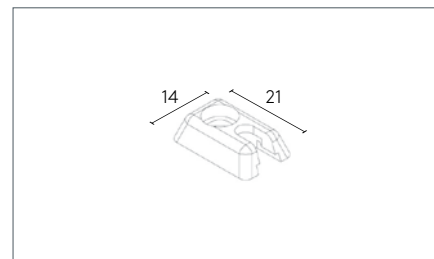
Spannfuß transparent (unten) Art. Nr. 15.6115
