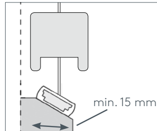
Schnitt Glasleiste mit Spanschuh und Unterschiene
