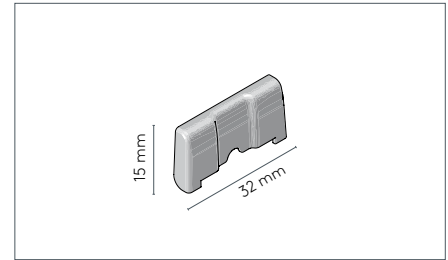
Abdeckung für Wandwinkel Art. Nr. 29.7825
