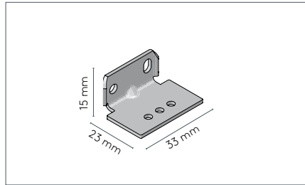
Wandwinkel Art. Nr. 29.7824
