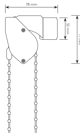
Querschnitt ISI-PIN mit Wandträger 65 mm
