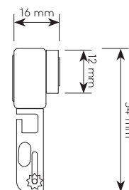
Querschnitt MINOR Wandclip 9750-04
