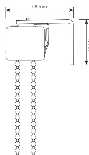
Querschnitt SMART mit Wandträger
