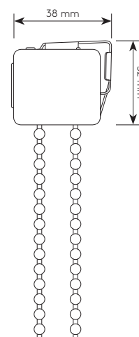
Querschnitt SMART mit Universalträger
