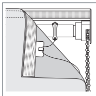
Technik ISI-CLICK mit Kettenbedienung
