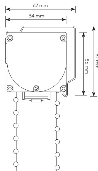
Querschnitt XL
