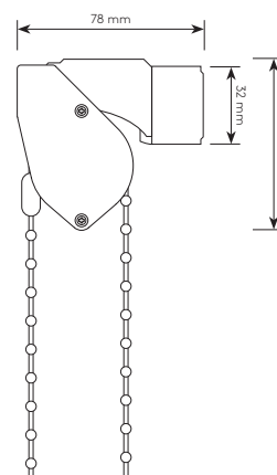
Querschnitt ISI-CLICK mit Wandträger 65 mm
