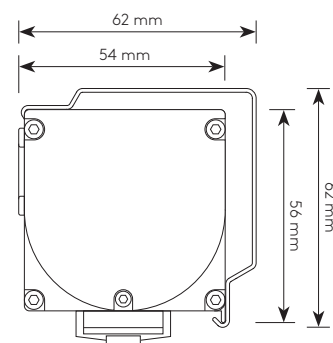
Querschnitt XL-EL mit Motor 230 V
