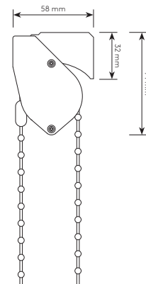
Querschnitt ISI-PIN mit Universalträger
