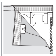
Technik ISI-PIN mit Kettenbedienung
