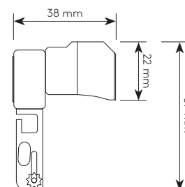
Querschnitt MINOR Universalträger 9210-10
