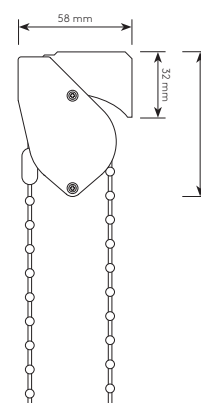
Querschnitt ISI-CLICK mit Universalträger
