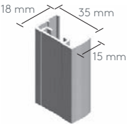
Detail Seitenschiene
