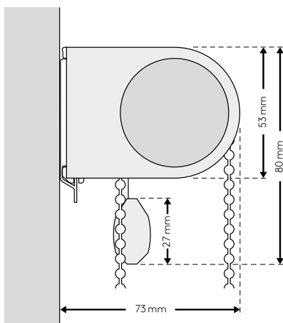
montáž na stěnu W
