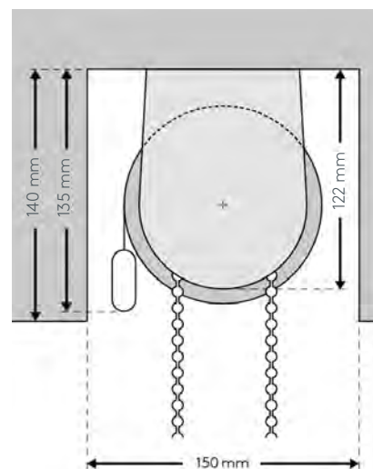
Montáž do šachty S
