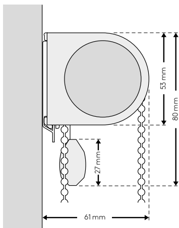
montáž na stěnu W
