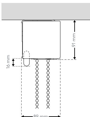
Montáž na strop D
