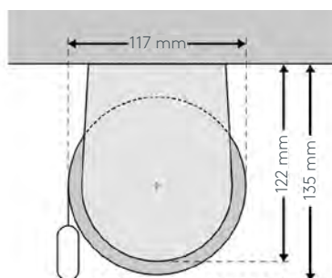
Montáž na strop D
