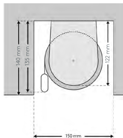
Montáž do šachty S
