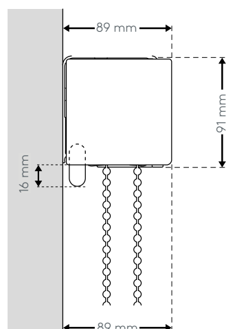
Montáž na stěnu W
