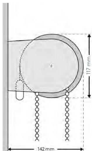
Montáž na stěnu W
