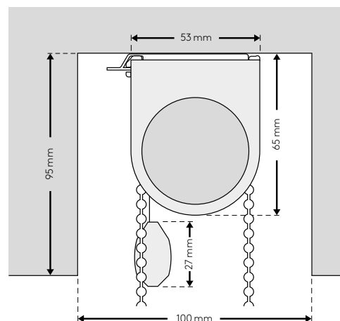
montáž do šachty S
