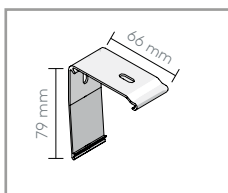
Univerzální držák 24.7511 pro stěnu a strop
