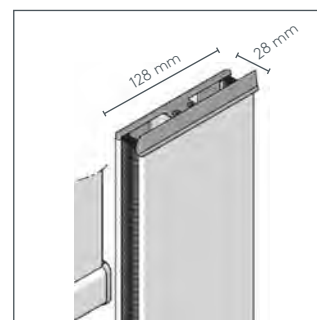
64 mm (spojené) látko a dolní profil jsou s bočním vedením
