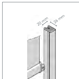
20 mm pouze dolní profil je s bočním vedením
