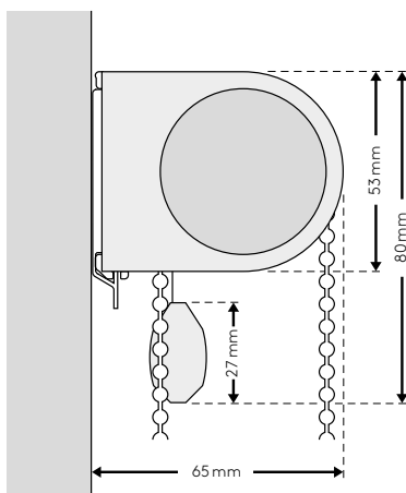
montáž na stěnu W
