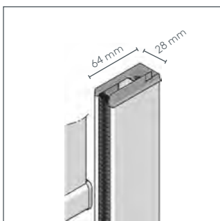
64 mm (standard) látko a dolní profil jsou s bočním vedením
