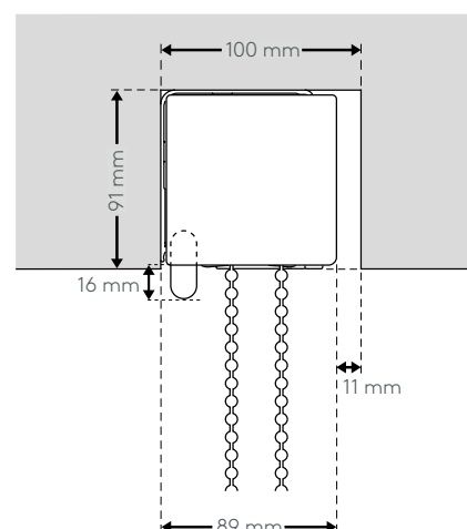
Montáž do šachty S
