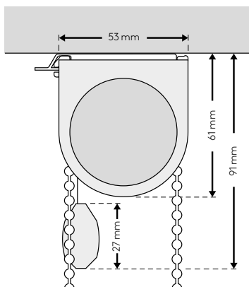
montáž na strop D
