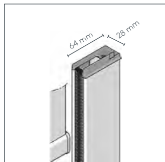
64 mm (standard) látka a dolní profil jsou s bočním vedením
