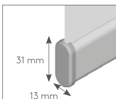
Dolní profil viditelný
