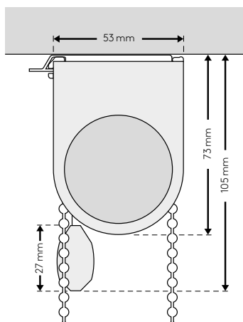
montáž na strop D
