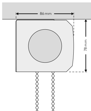
Montáž na stěnu W
