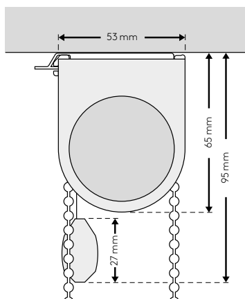
montáž na strop D
