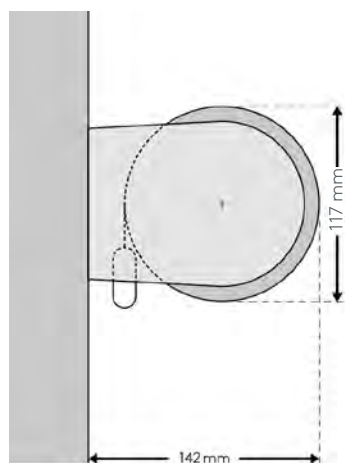
Montáž na stěnu W
