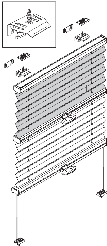
Reihenfolge Schienenmontage
