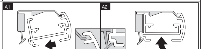
Reihenfolge Schiene einklippen
