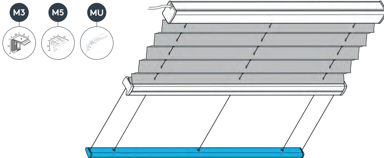
Abb. PLE2 Spanndrähte feststehend, Abstand ca. 20 cm.
