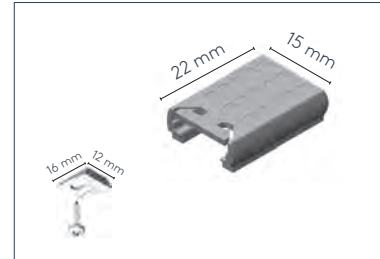
Spannschuh Art. Nr. 29.7941 bzw. 29.7943
