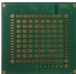
Figure 4. Actual Module (Bottom View)
