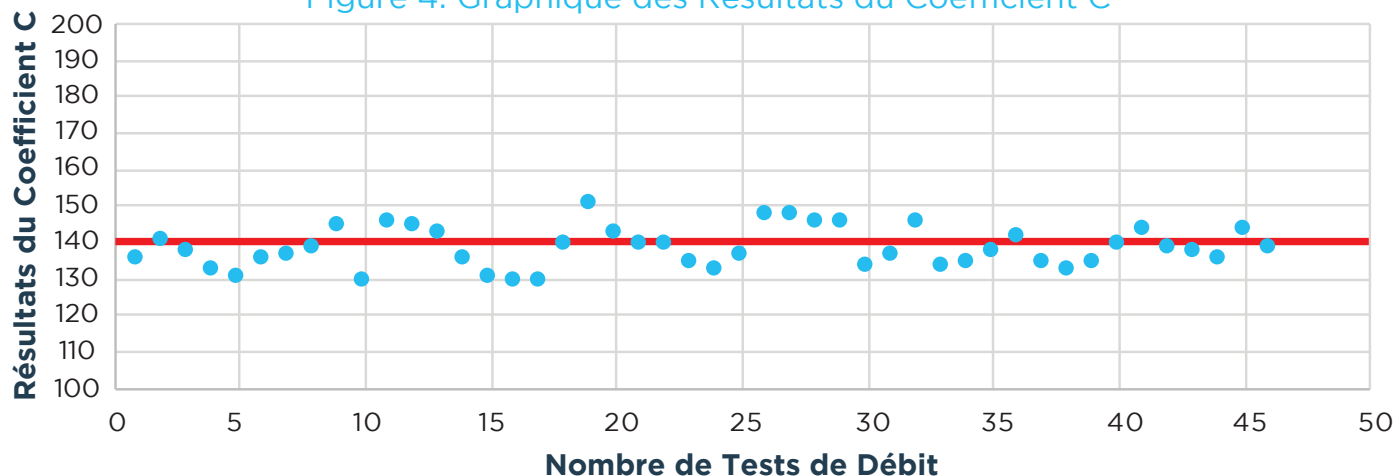
Figure 4: Résultats des tests de débit du Tableau 2 – la base du C de 140 pour les tuyaux en fonte ductile revêtus de mortier de ciment.
