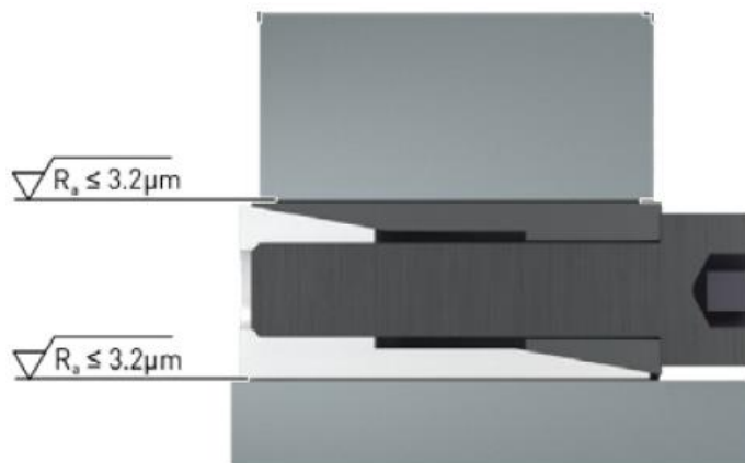
Bild 4-1 Passungszuordnung
