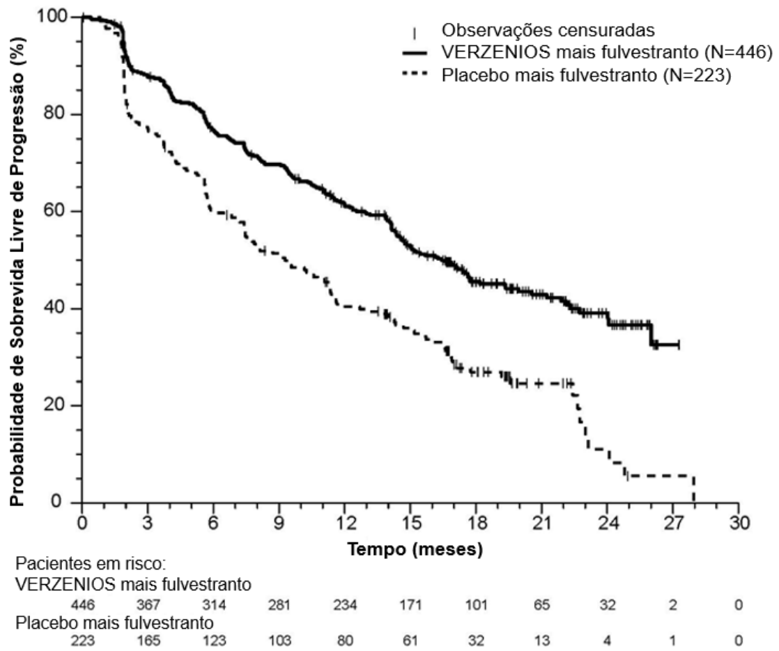
Figura 3: Curvas de Kaplan-Meier de Sobrevida Livre de Progressão: VERZENIOS mais fulvestranto versus Placebo mais fulvestranto (MONARCH 2)
