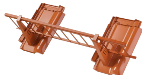
6 system przeciwnieęgowy
