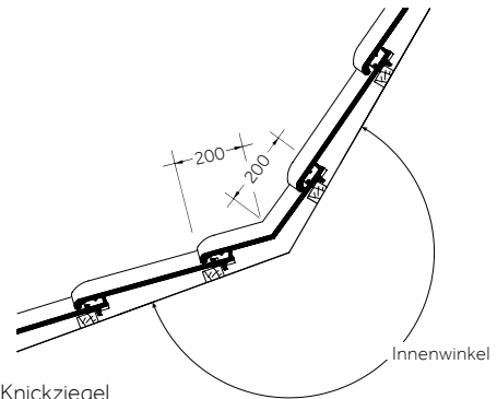
Knickziegel
