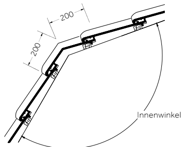
Mansardziegel
