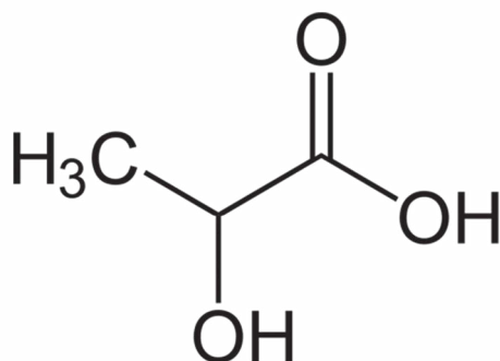
Milchsäuremolekül
