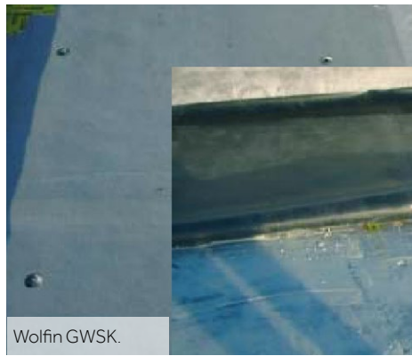
Wolfin GWSK auf einer kaschierten Zusatzdämmung.
