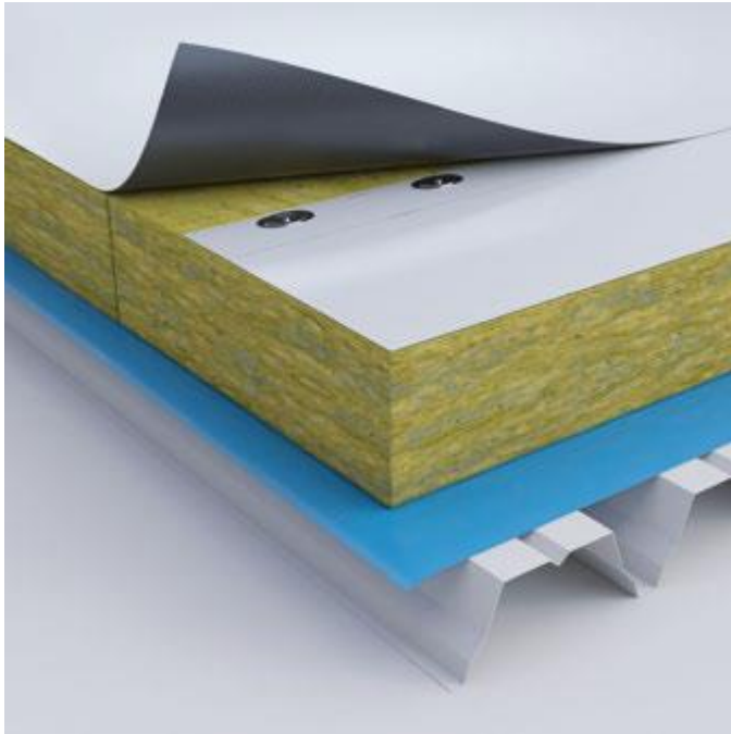
Foto 2.2 (Steinwolle-Dämmsystem auf Trapezblech)
