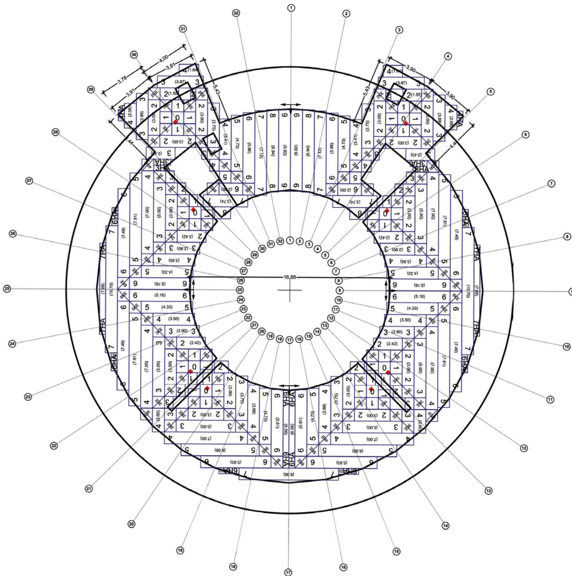
Beispielhafter Gefälleplan
