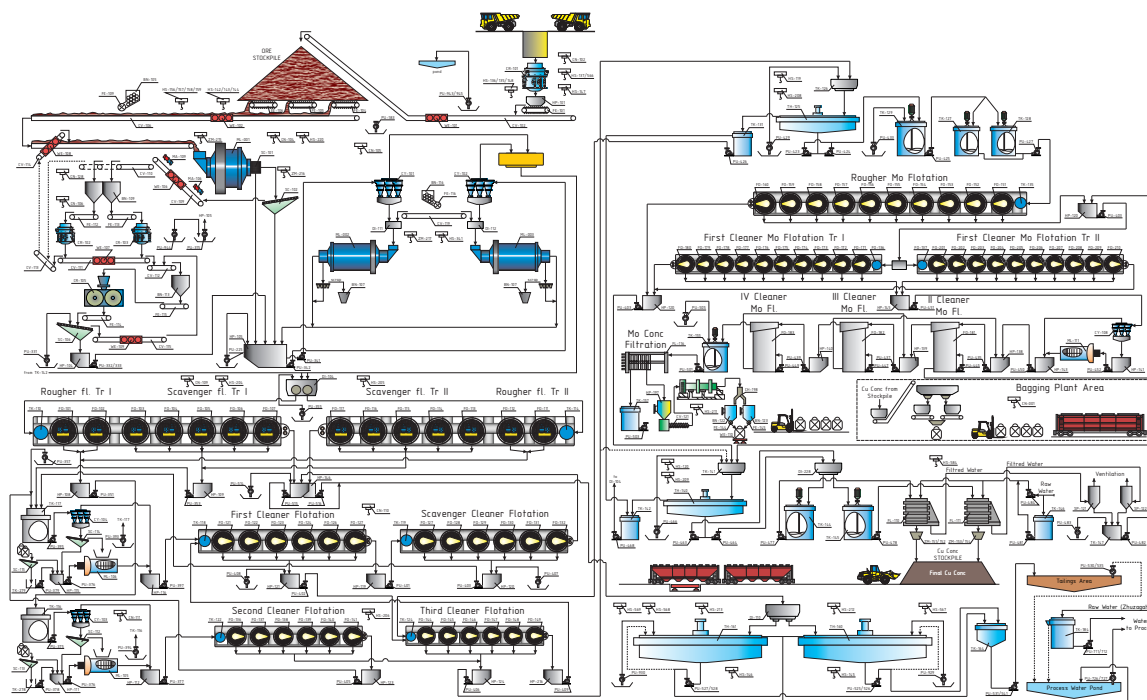
Figure 1 – Aktogay Flowsheet
