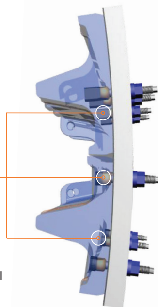
Aparafusamento MillSafe™
