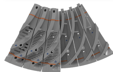
Bandas Guías de Ubicación MillSafe®
