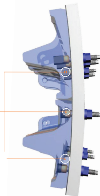
Система болтовых креплений MillSafe™
