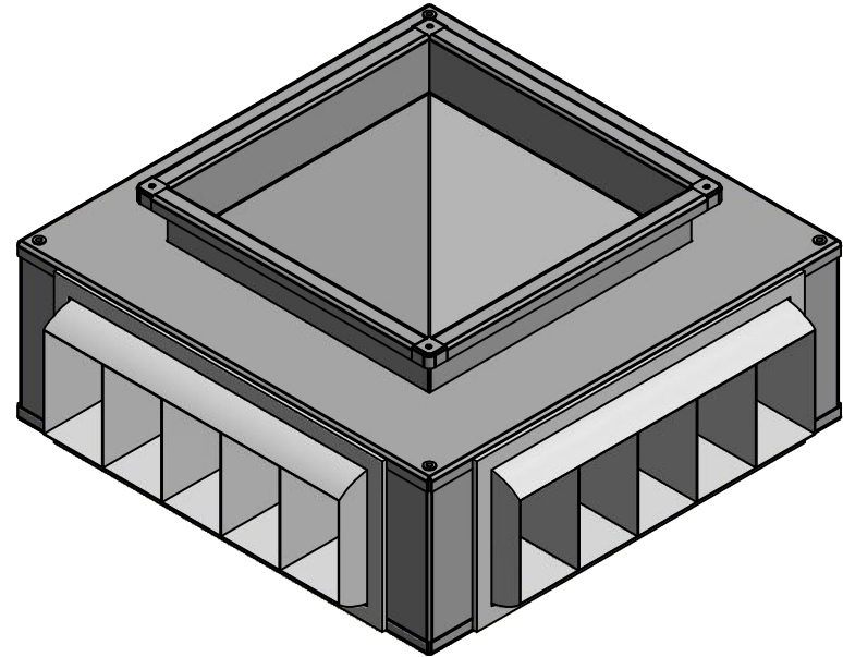
DRUM LOUVER PLENUM-DIFFUSER
