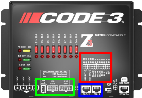
Z3 INPUT WIRES
