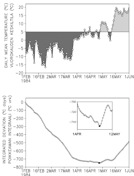
Kuva 4. Kasvukauden alkamisajankohdan määrittäminen lämpötilaerotusmenetelmää käyttäen. Ylempi kuva esittää lämpötilan vuorokausikeskiarvoja pisteessä 62.125°N, 26.125°E vuoden 1984 helmikuusta toukokuuhun. Lämpötilojen poikkeamat 5°C rajalämpötilasta alaspäin ja ylöspäin on varjostettu tummalla ja vaalealla harmaasävyillä. Alakuva: Kuhunkin päivään mennessä kertynyt vuorokausikeskilämpötilojen poikkeamien summa laskettuna helmikuun 1. päivästä lähtien. Tämän summalausekkeen minimiarvo, joka saavutettiin huhtikuun 27. päivänä, on merkitty käyrälle mustalla ympyrällä. Pikku kuva esittää suurennettuna lämpötilapoikkeamien summalausekkeen arvoja aikavälillä 1.4.–12.5.
