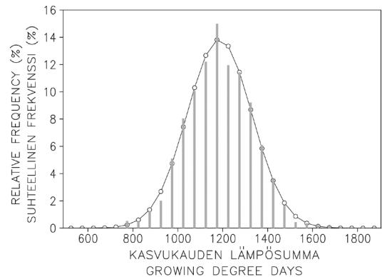
Kuva 8. Kasvukauden lämpösommen frekvenssijakauma pisteessä 62.125°N, 26.125°E jakson 1971–2000 ilmastossa (harmaat pylväät) sekä jakaumaan sovitettu normaalijakauma (musta käyrä). Jakauman keskiarvo on 1 186 ja keskihajonta 144 astepäivää. Frekvenssijakauma on muodostettu käymällä läpi kunkin 30 vuoden lämpösommat kaikista malliajoista.
