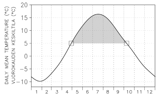
Kuva 3. Termisen kasvukauden alkamisen, päättymisen ja lämpösumman määrittäminen klimatologisen keskiarvomenetelmän avulla esimerkkipisteessä 62.125^{\circ}\text{N} , 26.125^{\circ}\text{E} jakson 1971–2000 lämpötilatietojen perusteella. Käyrä esittää kullekin vuoden päivälle (1.1.–31.12.) laskettua tuon ajanjakson ilmastoa kuvaavaa pitkäaikaisista keskilämpötilaa. Viiden asteen rajan ylitys keväällä ja alitus syksyllä (termisen kasvukauden alku ja päättyminen) on merkitty kuvaan neliöillä ja kasvukauden aikana kertynyt lämpösumma harmaalla varjostuksella.
