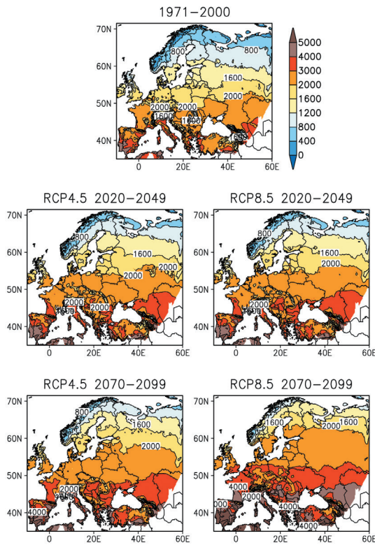
Kuva 7. Keskimääräinen kasvukauden lämpösomma (astepäivinä) Euroopassa vuosina 1971–2000 (yläkuva) sekä mallitulosten keskiarvoon perustuvat arviot jaksoille 2020–2049 (keskimmäinen rivi) ja 2070–2099 (alarivi), erikseen RCP4.5- (vasemmalla) ja RCP8.5-skenaarioille (oikealla). Samanarvonkäyrien väli on 2 000 astepäivään asti 400, suuremmilla arvoilla 1 000.
