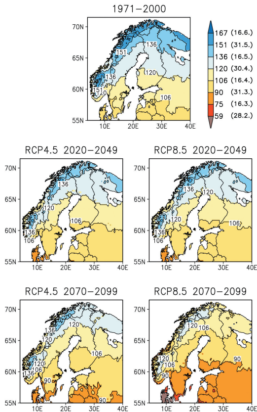
Kuva 5. Termisen kasvukauden keskimääräinen alkamispäivä Pohjois-Euroopassa vuosina 1971–2000 (yläkuva) sekä mallitulosten keskiarvoon perustuvat arviot alkamisajankohdalle jaksojen 2020–2049 (keskimmäinen rivi) ja 2070–2099 (alarivi) aikana; arviot on annettu erikseen RCP4.5- (vasemmalla) ja RCP8.5-skenaarioille (oikealla). Väritys ja samanarvonkäyrät ilmaisevat alkamishetken juoksevana päivämääränä vuoden alusta; esimerkiksi päivä numero 120 vastaa huhtikuun 30. päivää (ks. väriasteikon vieressä olevaa selitystä).
