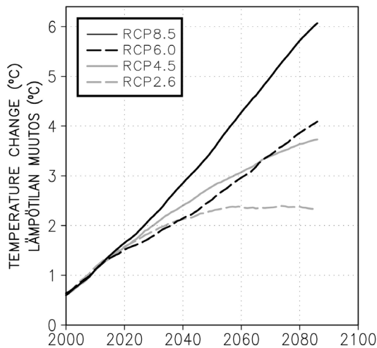
Kuva 1. Suomen vuotuisen keskilämpötilan muutos (°C) vuosina 2000–2085 verrattuna jakson 1971–2000 keskilämpötilaan; 28 ilmastomuutosmallin tulosten keskiarvoista laskettu 30 vuoden liukuva keskiarvo. Muutokset on annettu erikseen neljälle kasvihuonekaasuskenaariolle: RCP8.5, RCP6.0, RCP4.5 ja RCP2.6 (selitys kuvassa).
