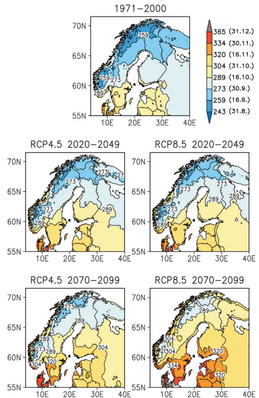
Kuva 6. Termisen kasvukauden keskimääräinen päättymisajankohta vuosina 1971–2000 (yläkuva) sekä mallitulosten keskiarvoon perustuvat arviot jaksoille 2020–2049 (keskimmäinen rivi) ja 2070–2099 (alarivi). Numerot ovat juoksevia päivämääriä vuoden alusta; esimerkiksi päivä numero 304 vastaa lokakuun 31. päivää (ks. selityspalkkia).
