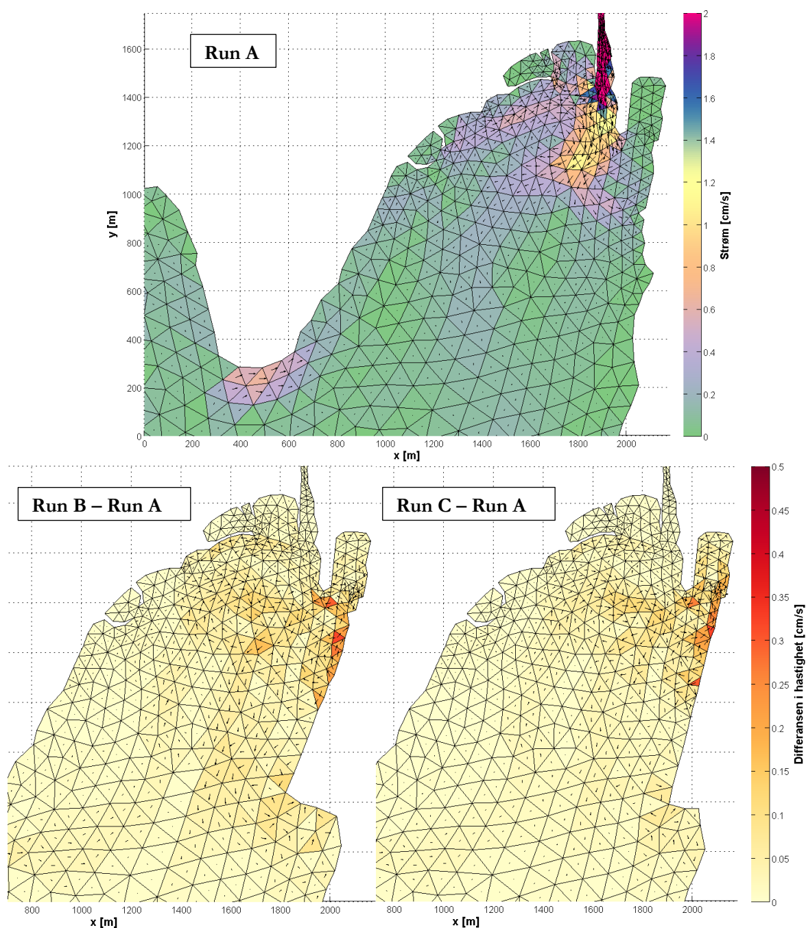
Figur 14. Strømfeltet ved høyvann i run A (øverst), samt strømmen i run B fratrasket strømmen i run A (nederst, venstre) og strømmen i run C fratrasket strømmen i run A (nederst, høyre)
