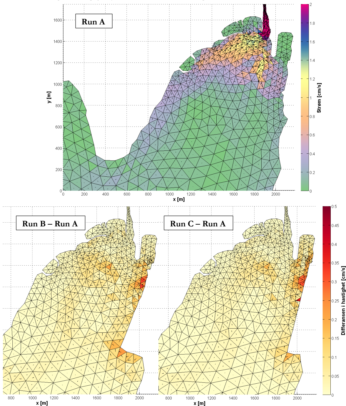
Figur 16. Strømfeltet ved lavvann i run A (øverst), samt strømmen i run B fratrasket strømmen i run A (nederst, venstre) og strømmen i run C fratrasket strømmen i run A (nederst, høyre)
