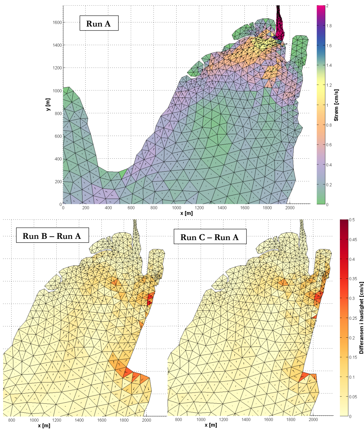
Figur 17. Strømfeltet ved stigende tidevann i run A (øverst), samt strømmen i run B fratrasket strømmen i run A (nederst, venstre) og strømmen i run C fratrasket strømmen i run A (nederst, høyre)
