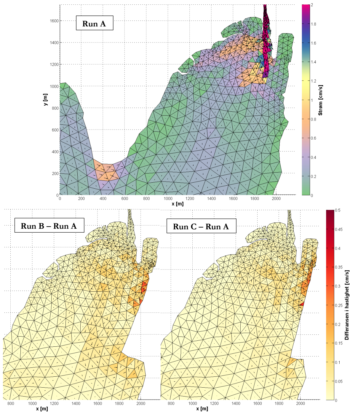
Figur 15. Strømfeltet ved synkende tidevann i run A (øverst), samt strømmen i run B fratrasket strømmen i run A (nederst, venstre) og strømmen i run C fratrasket strømmen i run A (nederst, høyre)
