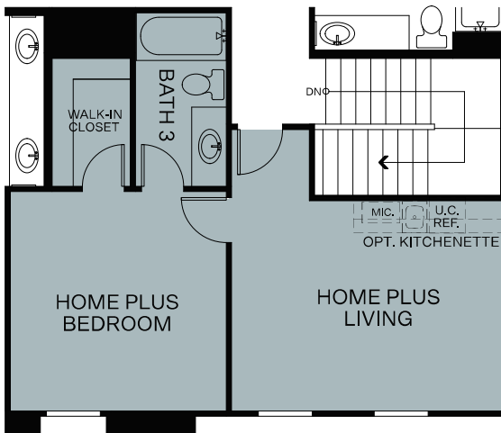
OPT. HOME PLUS SUITE ILO LOFT
