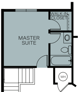
OPT. MASTER SUITE ADDS: 233 SQ.FT.
