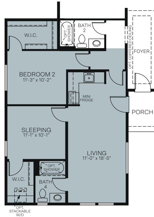
OPTIONAL HOME PLUS
