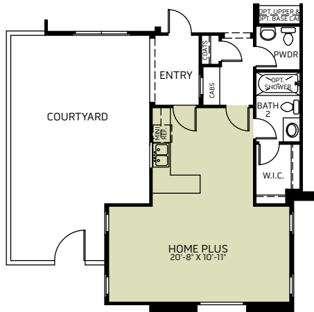
OPTIONAL HOME PLUS
