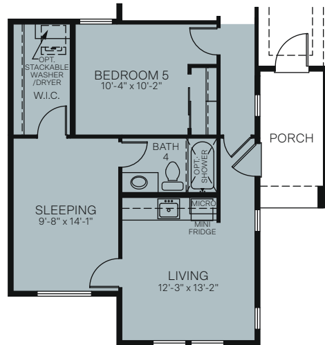
OPTIONAL HOME PLUS
