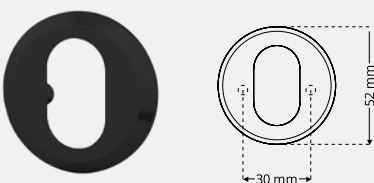
Cylinderring DR 8320
