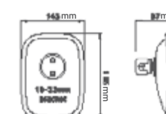
7121-321 (Flat) 7120-321 (Convex)
