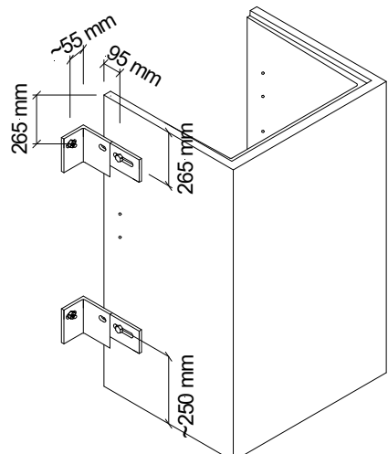
Bild 22: Lichtschacht mit 4 Befestigungswinkel Typ KOMBI A, ISO 20 oder 30 unten und oben
