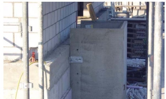
Bild 36: Befestigungswinkel Typ KLEIN
