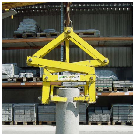
Versetzzange für Transport von Palisaden
