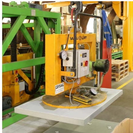
Vakuum Verlegegerät VACU LIFT bis 1600 kg
