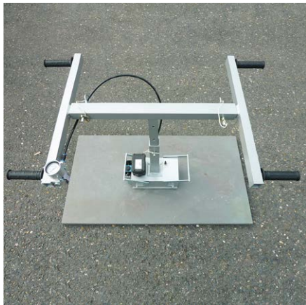
BETA Akku Vakuumversetzgerät bis 150 kg
