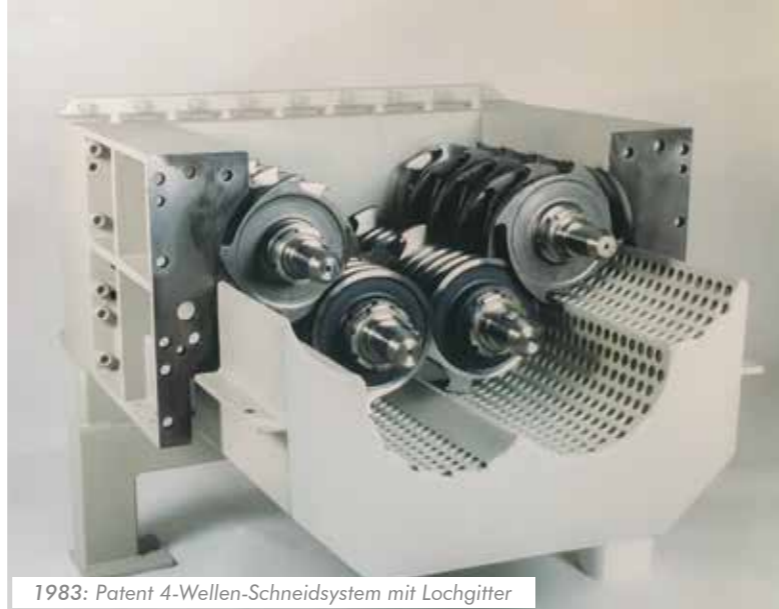
1983: Patent 4-Wellen-Schneidsystem mit Lochgitter
